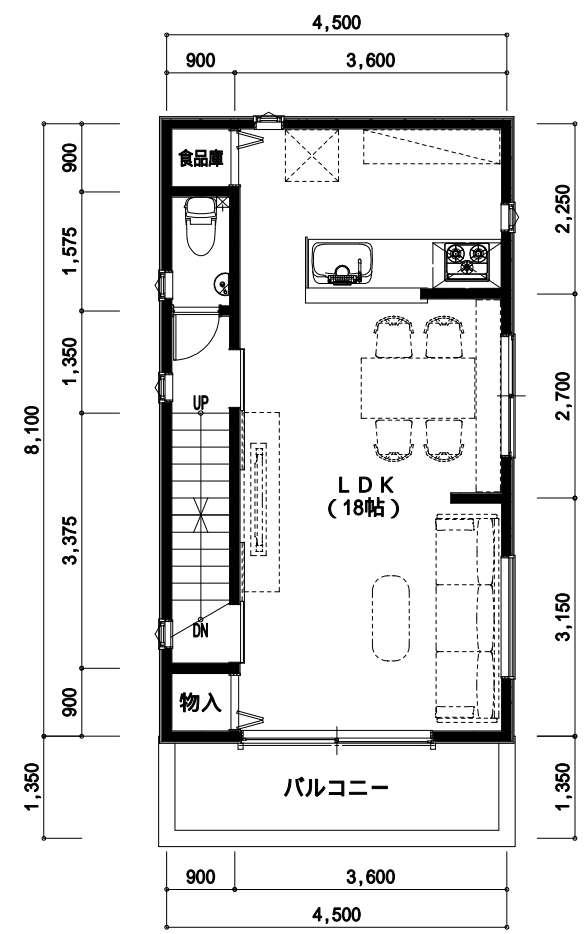
2階 平面図
