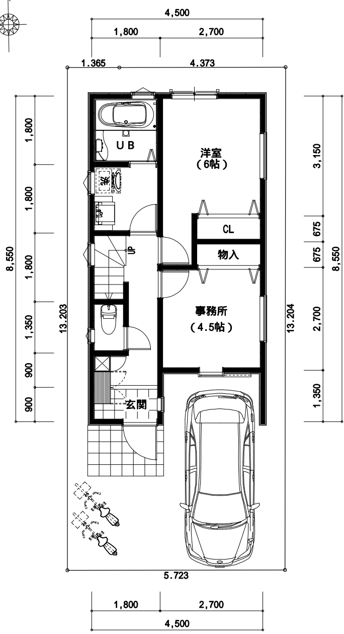
1階 平面図
