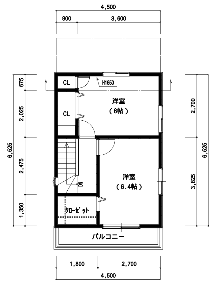
3階 平面図
